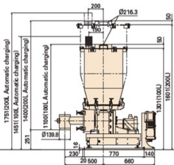
CE-R-4D-MP(200L)
